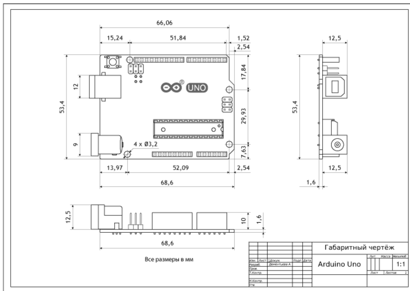
Modèle solidWorks carte Arduino UNO R3
